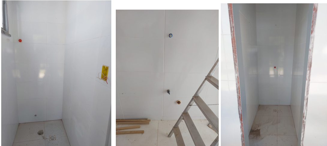
Fotos 03. Instalação de registros, pontos de esgoto, pontos de água fria, ralos
