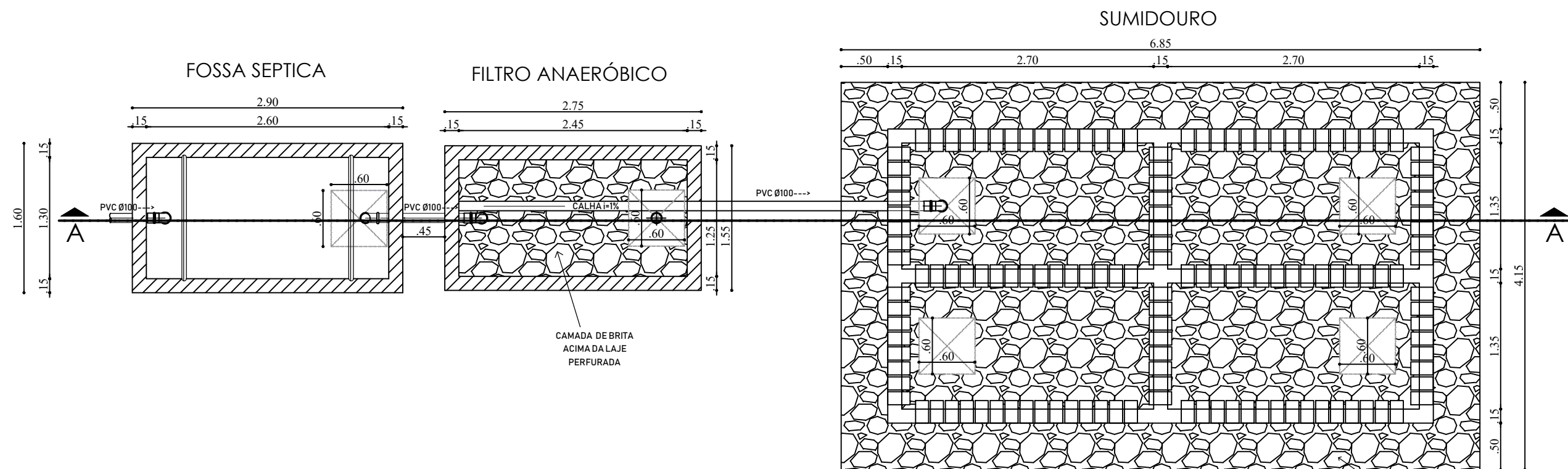
PLANTA BAIXA ESCALA 1:50
