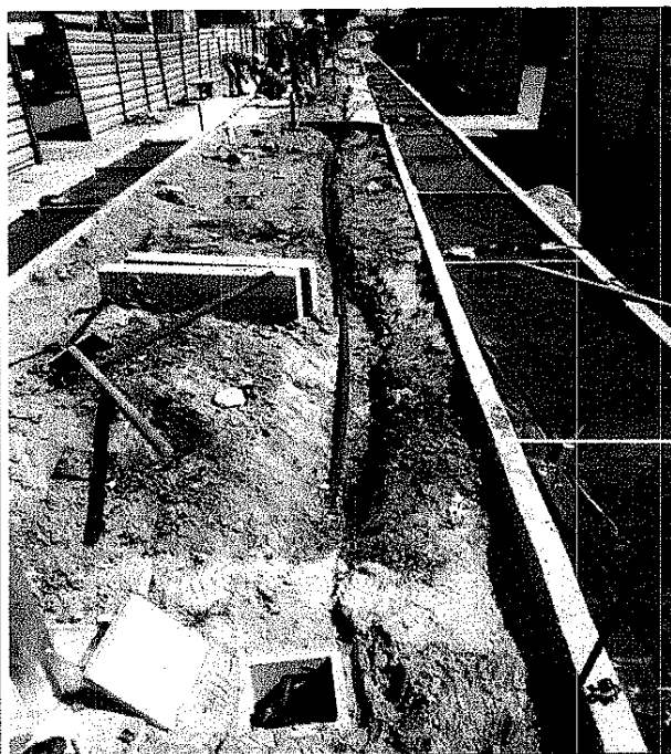
Foto 02: Escavação de vala, instalação de eletroduto e caixa de derivação.
