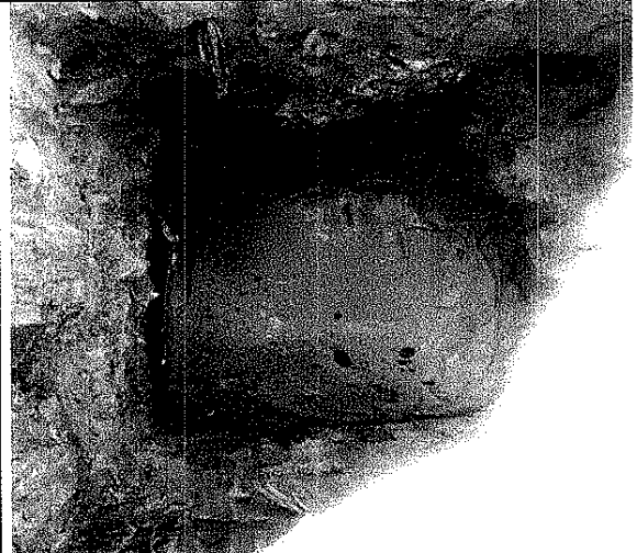
Foto 06: Adequação para maior estabilidade da sapata dos postes, aplicando lona plástica e o concreto magro.
